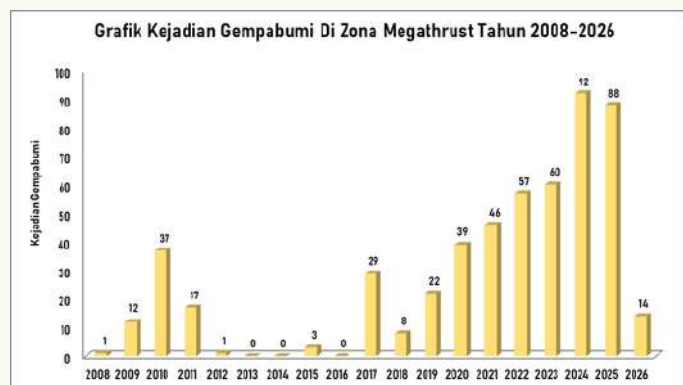
Gambar 19. Distribusi Kejadian Gempabumi Zona Megathrust Oktober 2008 – Februari 2026
