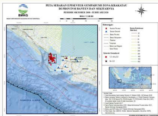
Gambar 16. Peta Sebaran Episenter Gempabumi Zona Krakatau Oktober 2008 – Februari 2026
