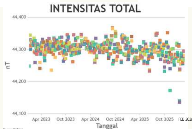
Gambar 24. Grafik nilai Inklinasi, Deklinasi dan Intensitas Total Bulan April 2023 – Februari 2026
