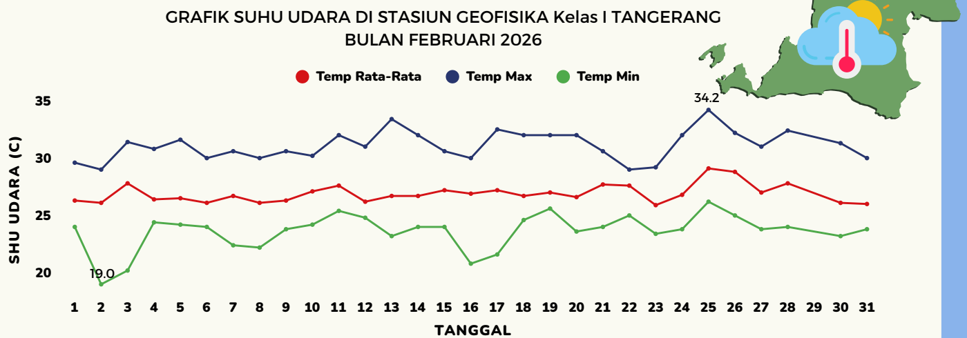
Gambar 26. Grafik Suhu Udara bulan Februari 2026
