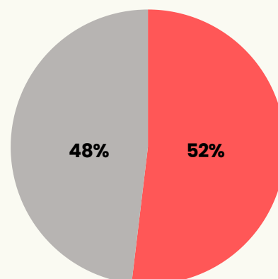
Gambar 4. Diagram persentase gempabumi berdasarkan lokasi gempa bulan Februari 2026
