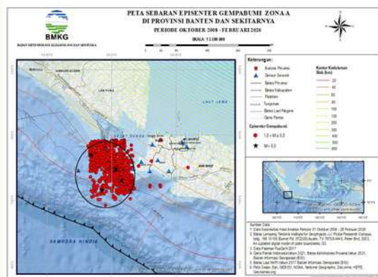
Gambar 9. Peta Sebaran Episenter Gempabumi Zona A Oktober 2008 – Februari 2026
