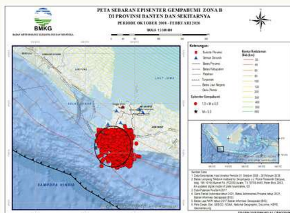
Gambar 11. Peta Sebaran Episenter Gempabumi Zona B Oktober 2008 – Februari 2026
