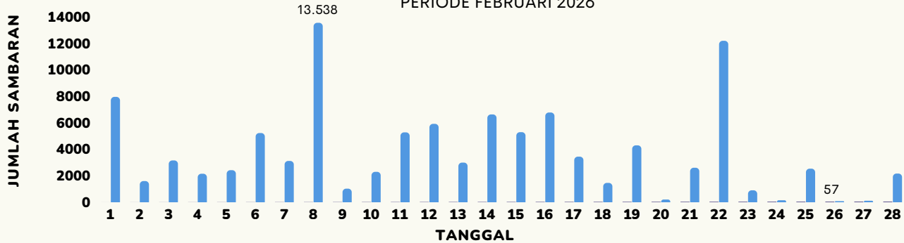
Gambar 22. Grafik frekuensi sambaran petir bulan Februari 2026
