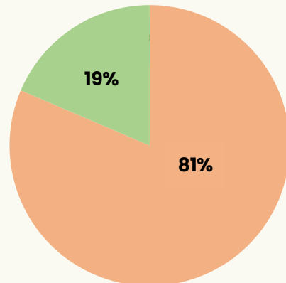
Gambar 2. Diagram persentase gempabumi berdasarkan magnitudo bulan Februari 2026
