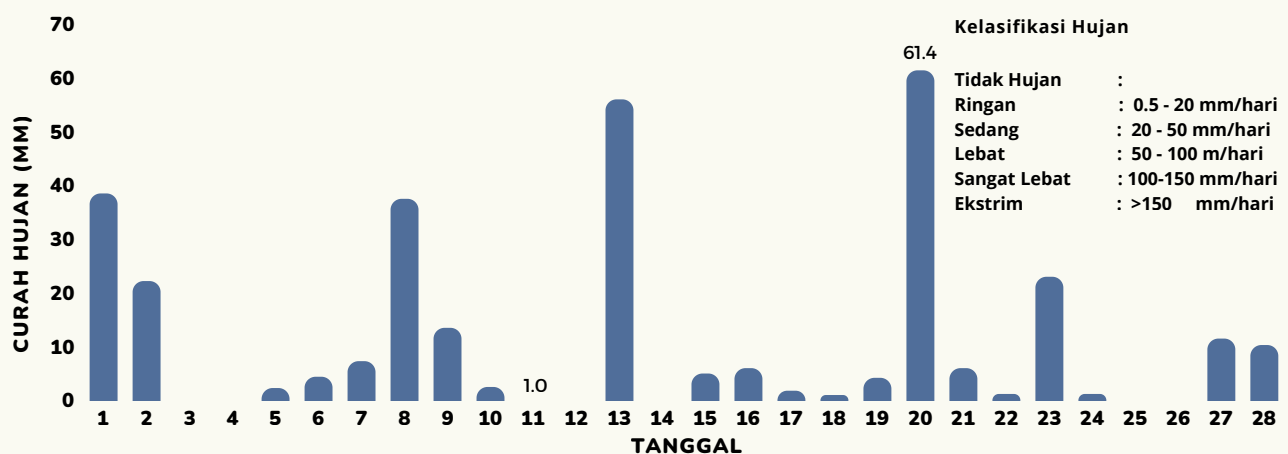
Gambar 25. Grafik Curah Hujan Harian bulan Februari 2026
