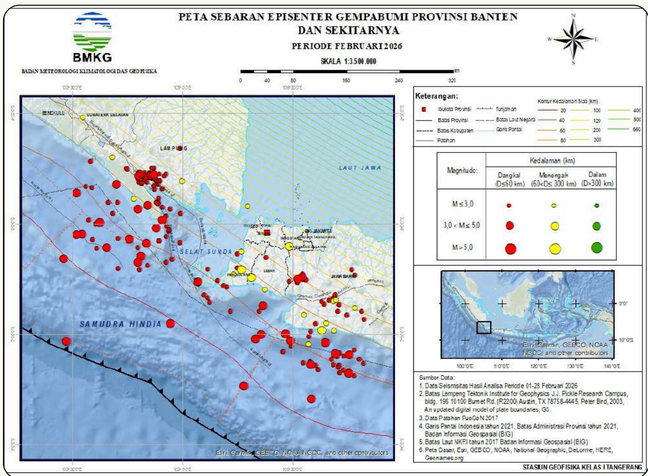
Gambar 1. Peta Sebaran Gempabumi di Wilayah Banten dan Sekitarnya bulan Februari 2026
