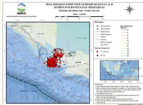
Gambar 13. Peta Sebaran Episenter Gempabumi Zona C dan D Oktober 2008 – Februari 2026
