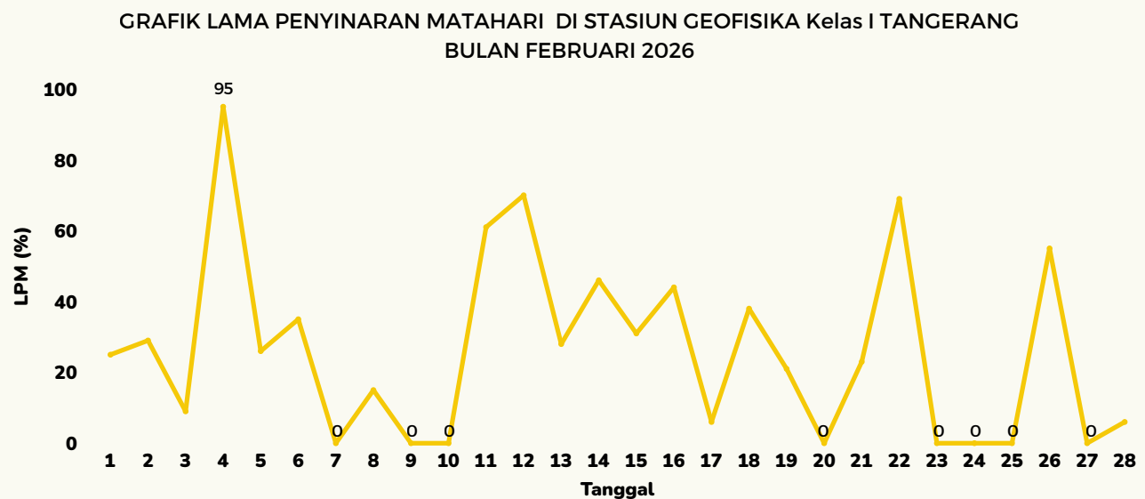
Gambar 27. Grafik Lama Penyinaran Matahari bulan Februari 2026
