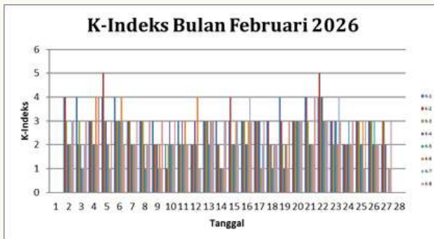
Gambar 24. Grafik nilai K-Indeks bulan Februari 2026
