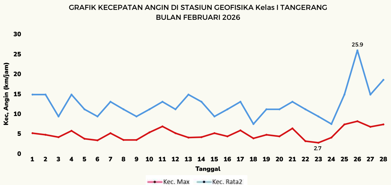
Gambar 29. Grafik Kecepatan Angin bulan Februari 2026
