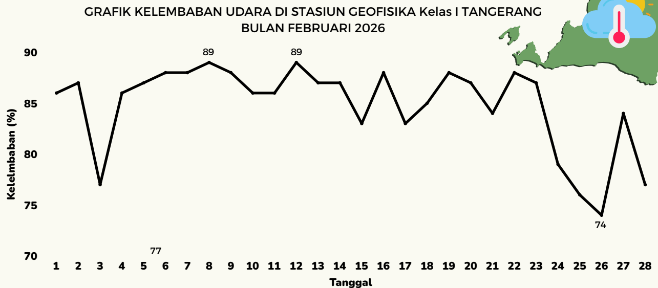
Gambar 28. Grafik Kelembaban Udara Rata-Rata bulan Februari 2026
