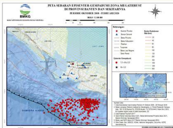
Gambar 18. Peta Sebaran Episenter Gempabumi Zona Megathrust Oktober 2008 – Februari 2026
