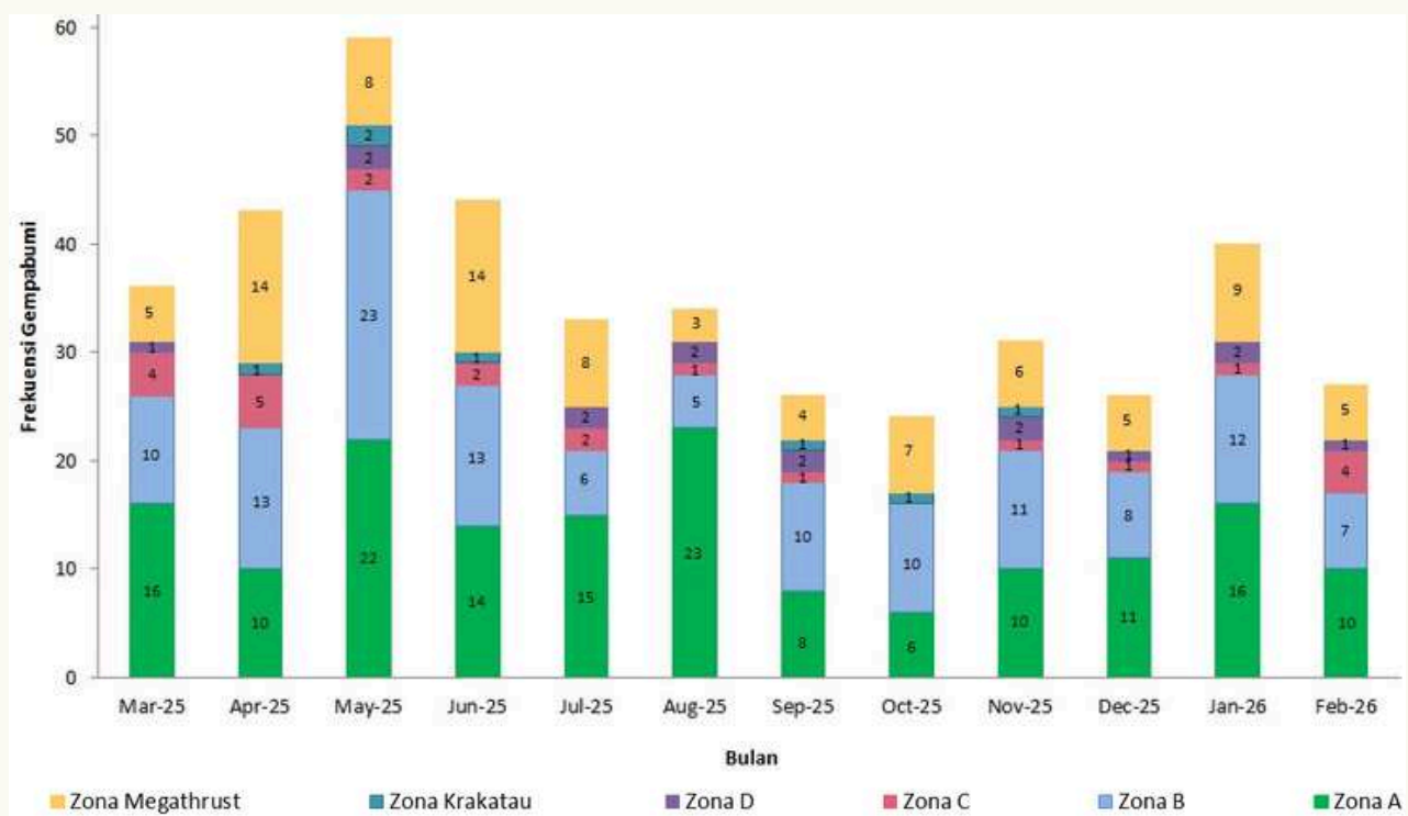
Gambar 21. Grafik Frekuensi Kegempaan di Enam Zona Periode Maret 2025 - Februari 2026
