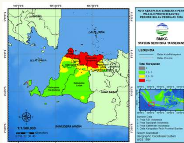
Gambar 23. Peta kerapatan sambaran petir Februari 2026
