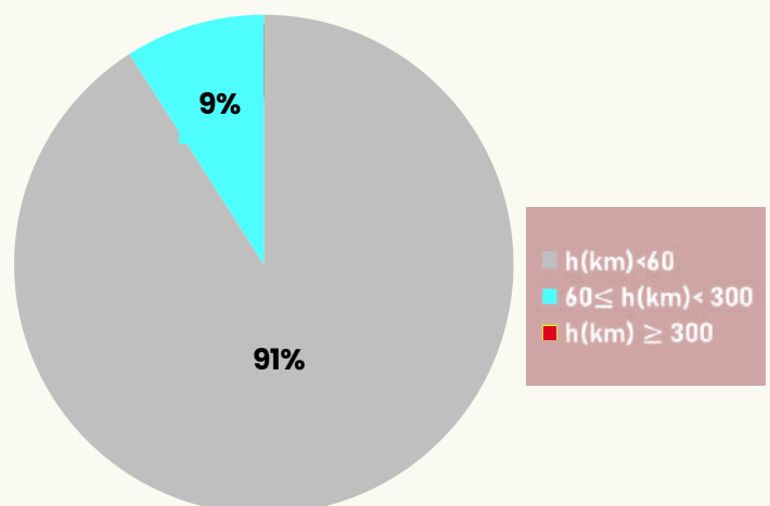
Gambar 2. Diagram persentase gempabumi berdasarkan kedalaman bulan Februari 2026
