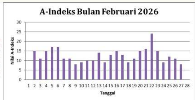
Gambar 25. Grafik nilai A-Indeks bulan Februari 2026
