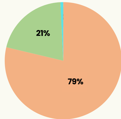
Gambar 2. Diagram persentase gempabumi berdasarkan magnitudo bulan April 2026
