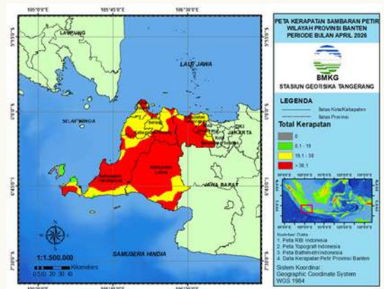
Gambar 23. Peta kerapatan sambaran petir April 2026
