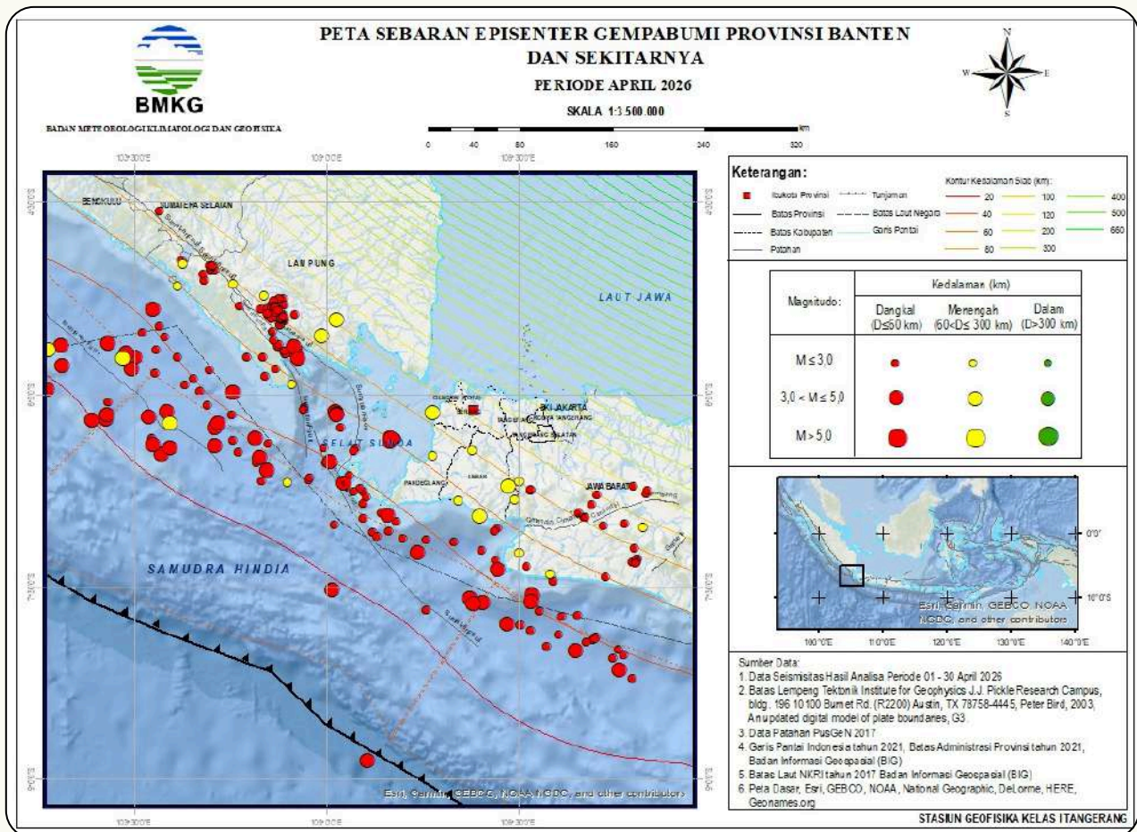
Gambar 1. Peta Sebaran Gempabumi di Wilayah Banten dan Sekitarnya bulan April 2026
