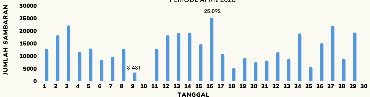
Gambar 22. Grafik frekuensi sambaran petir bulan April 2026
