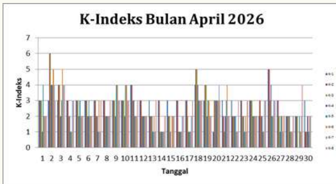
Gambar 24. Grafik nilai K-Indeks bulan April 2026
