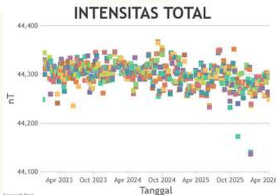
Gambar 24. Grafik nilai Inklinasi, Deklinasi dan Intensitas Total Bulan 2023 - April 2026
