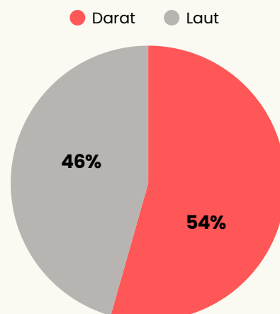
Gambar 4. Diagram persentase gempabumi berdasarkan lokasi gempa bulan April 2026
