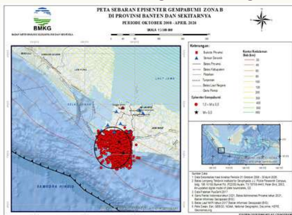
Gambar 11. Peta Sebaran Episenter Gempabumi Zona B Oktober 2008 – April 2026
