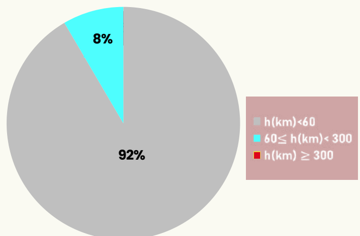
Gambar 2. Diagram persentase gempabumi berdasarkan kedalaman bulan April 2026
