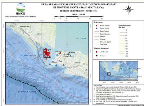
Gambar 16. Peta Sebaran Episenter Gempabumi Zona Krakatau Oktober 2008 – April 2026
