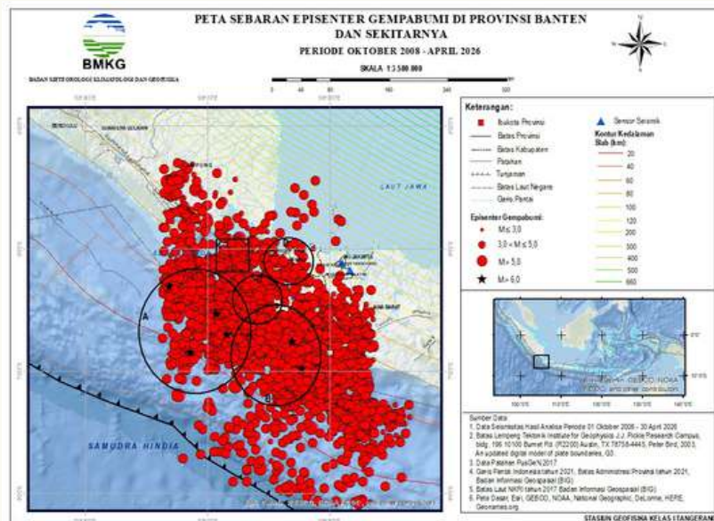
Gambar 8. Peta Sebaran Zona Episentris Gempabumi Di Provinsi Banten Tahun 2008 – April 2026
