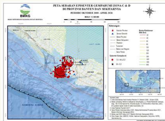
Gambar 13. Peta Sebaran Episentier Gempabumi Zona C dan D Oktober 2008 – April 2026
